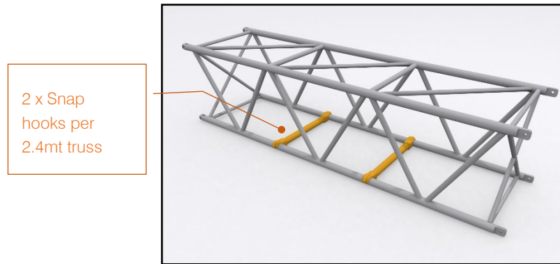
Fig. 46 - Maxibeam Snap Braces (24.4.1)
