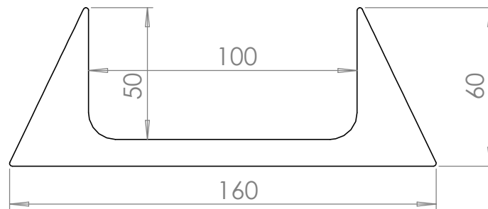
Profile 1:2
