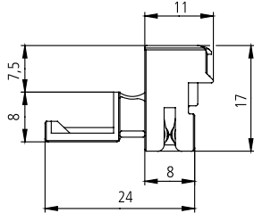
Darstellung endmontiert Designation final-assembled
