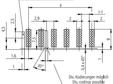
Div. Rastfenster möglich Div. lock windows possible
