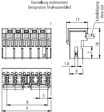
Darstellung endmontiert Designation final-assembled
