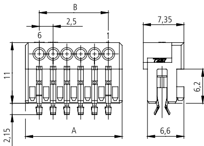
Darstellung vormontiert Designation pre-assembled
