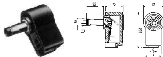
MP-202L RIGHT ANGLE
